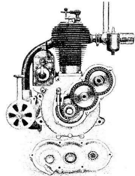
Interno e disposizione del Cambio di Velocità (brevettato)
