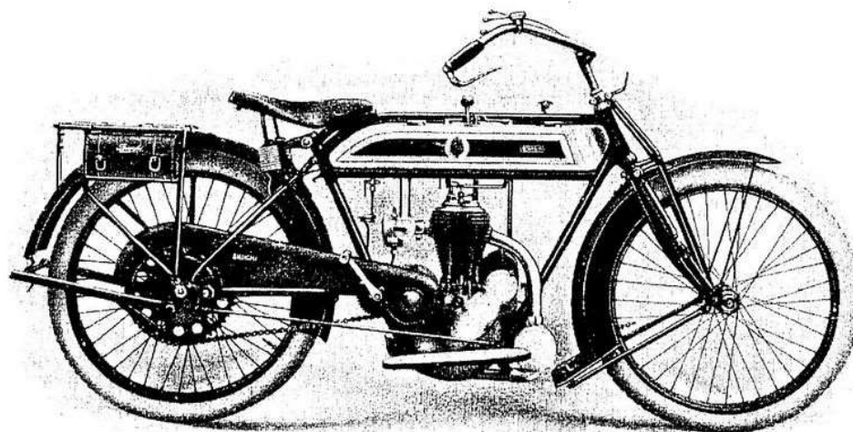
MOTOCICLETTA «BIANCHI» 3 1/2 HP - TIPO B
