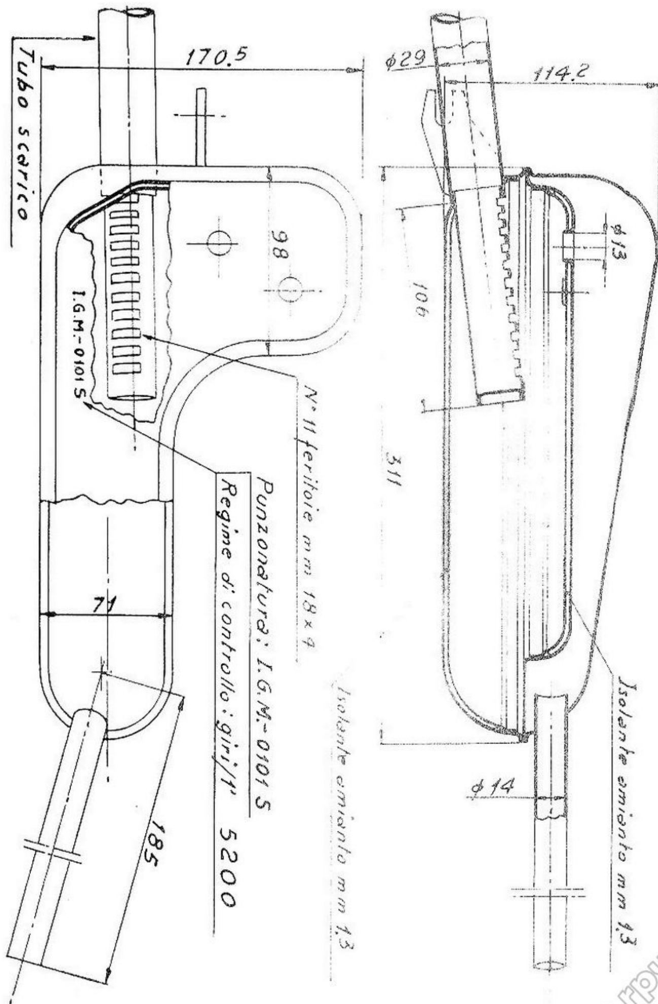
Silenziatore
