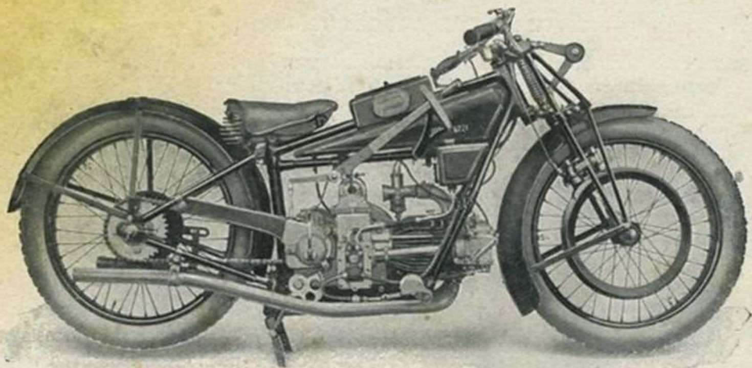
TIPO CORSA 4 V. Campionato d'Europa - lato distribuzione.
