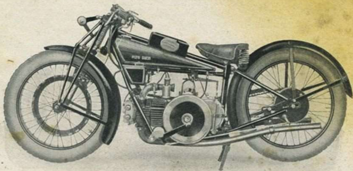
TIPO CORSA 4 V. Campionato d'Europa - lato volante.
