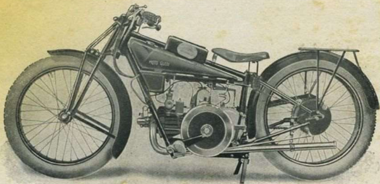
TIPO SPORT - lato volante.
