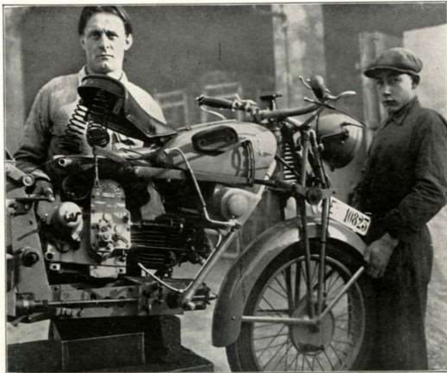
Fig. 18 - Vista del telaio aperto. Come si toglie il motore.
