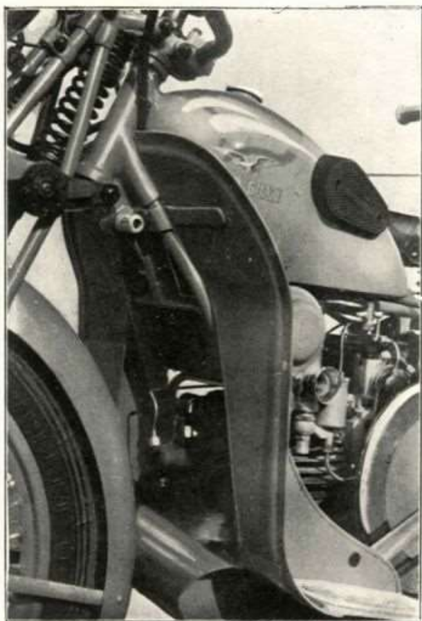
Fig. 9 - Gruppo sterzo - Pedane Scatola coprimolle.
