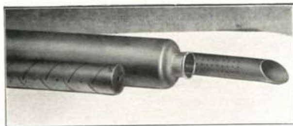
Fig. 69 - Come è formato il silenziatore del motociclo 32.
