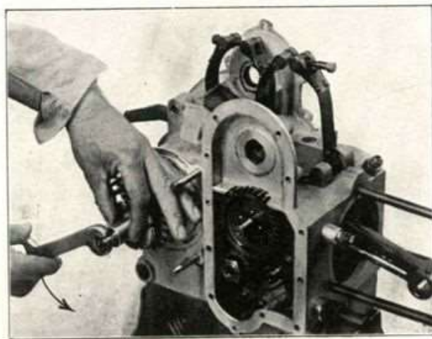
Fig. 42 - Come si leva l'asta interna di comando frizione.
