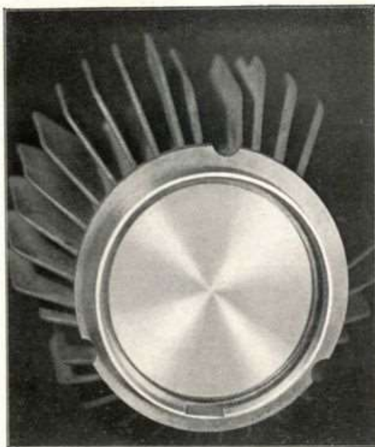
Fig. - 55 La figura mostra come si eseguisce la verifica dei segmenti nel cilindro.
