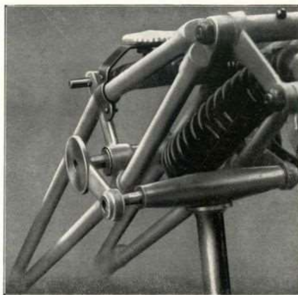
Fig. 37 - Come si leva il biscottino sinistro.
