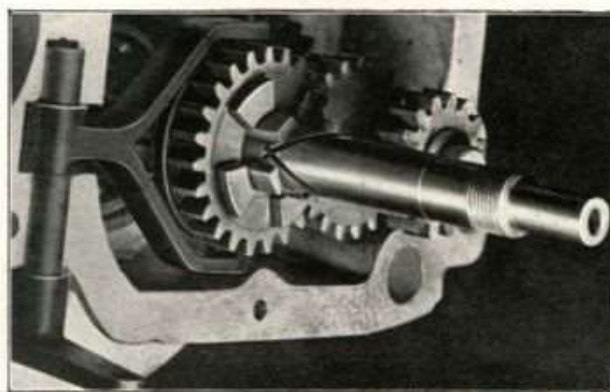
Fig. 64 - La figura mostra l'ingranaggio scorrevole montato sul primario del cambio e forcella con forcellino di ricambio.
