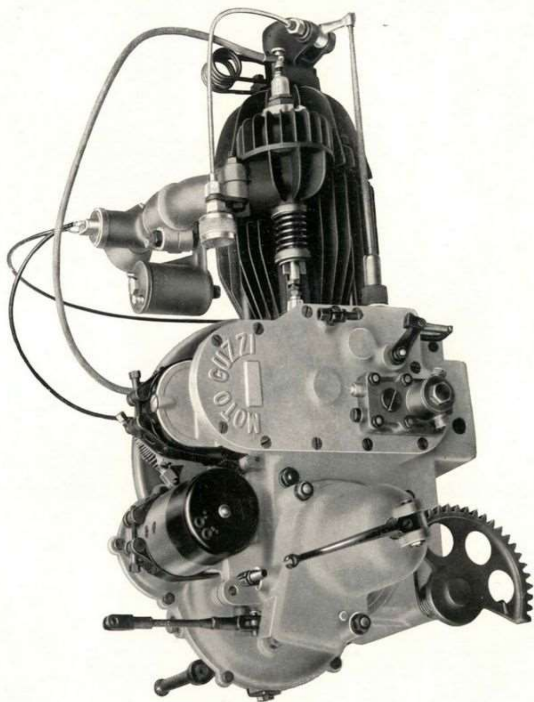
Fig. 1 - Gruppo motore cambio, lato distribuzione
