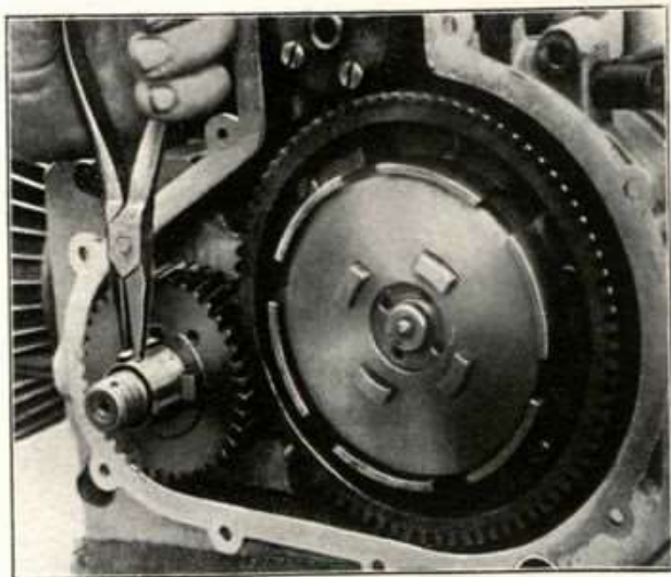
Fig. 41 - Levare la chiavella prima di sfilare il pignone motore.
