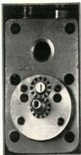
Fig. 71 - Il corpo pompa visto dall'interno. È visibile la pompa di mandata a ingranaggi.
