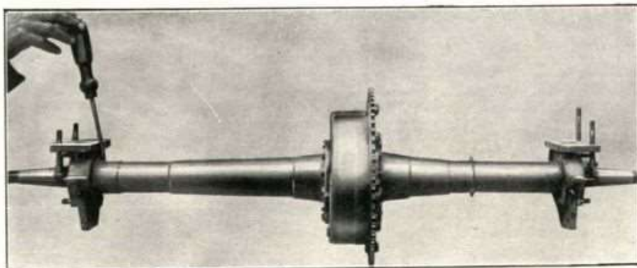
Fig. 102 - Come si leva la vite di fermo dei para acqua. Quello di destra è già stato spostato verso il centro.
