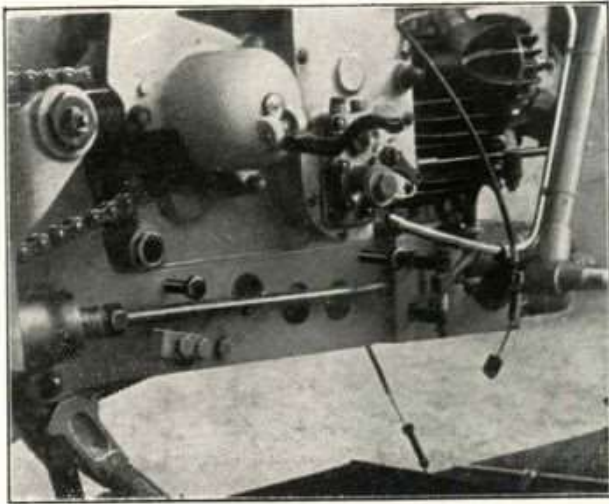
Fig. 16 - Sono visibili i due bulloni che fissano inferiormente il carter alle piastre porta motore.
