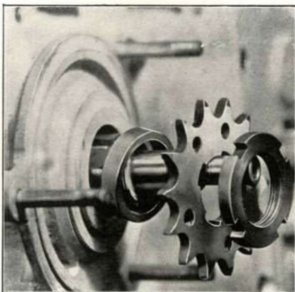
Fig. 45 - Come, dopo allentata la ghiera di serraggio, si levano il pignone e l'anello spessore.
