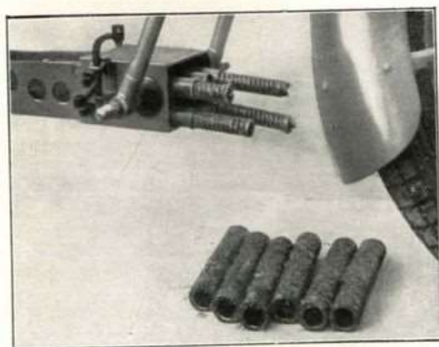
Fig. 22 - Le 6 molle esterne sono già tolte. Si vedono le molle interne parzialmente sfilate.
