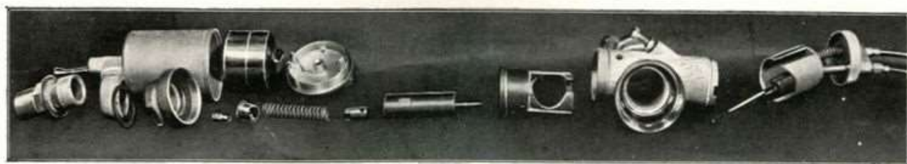
Fig. 67 - Il carburatore smontato.
