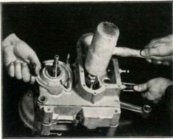
Fig. 46 - Come si apre il carter. Tenendolo sospeso con le mani e battendo alternativamente sull'estremità dell'albero a gomito...
