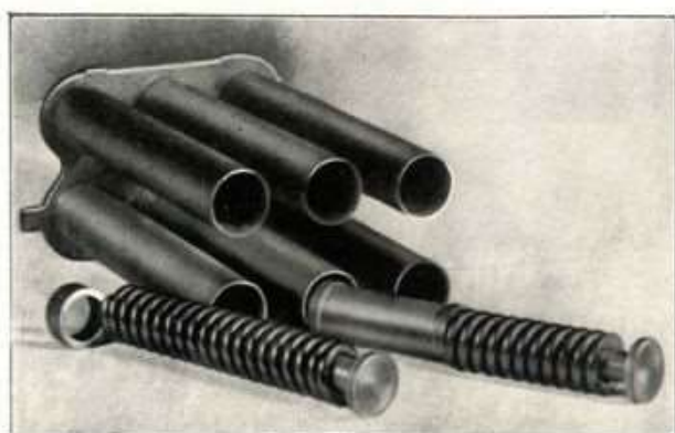
Fig. 83 - Moto monoposto. Si notino la vera spessore, la molla e la bussoletta di pressione laterali (a sinistra) e centrali.
