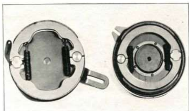
Fig. 89 - Piatto portaceppi posteriore e anteriore.
