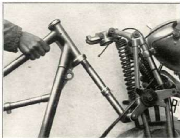
Fig. 30 - Come si sfila il canotto di guida dal canotto del telaio (pipa di sterzo).
