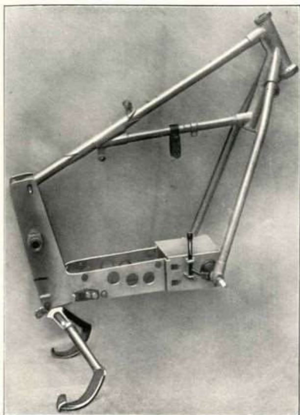
Fig. 31 - Vista del telaio centrale.
