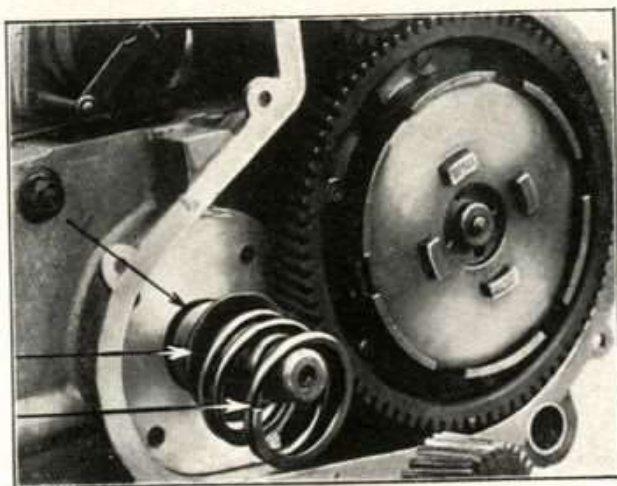
Fig. 40 - Come, tolto il pignone motore, si sfilano le molle di spinta, le ranelle di appoggio e la ranella premistoppa.
