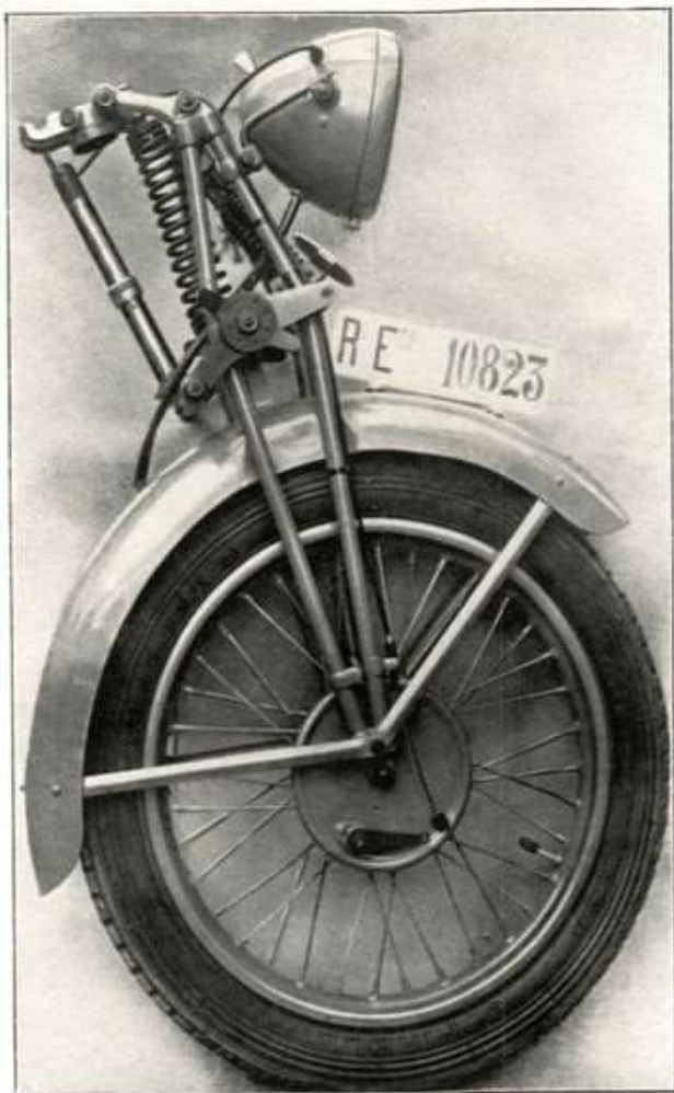
Fig. 33 - Gruppo forcella anteriore completo.
