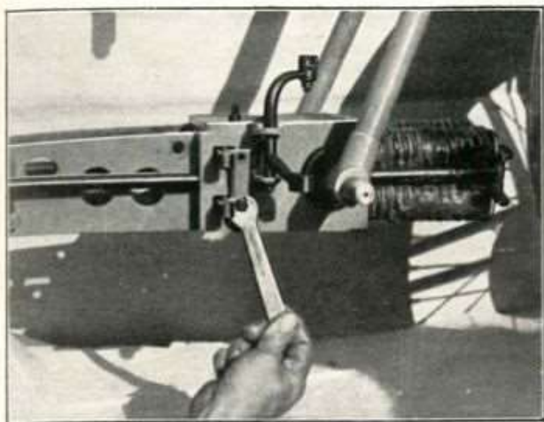
Fig. 25 - Come si leva la piastrina di fermo delle cremagliere.
