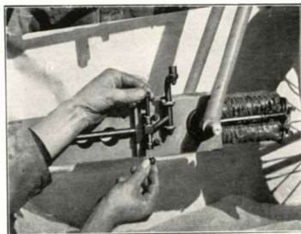
Fig. 24 - Come si leva la vite di tenuta (verticale) delle cremagliere.
