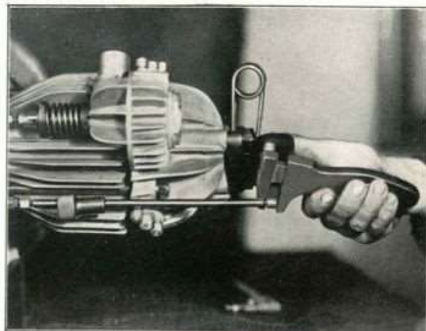
Fig. 76 - Come si monta l'asta di comando per bilancere di scarico.
