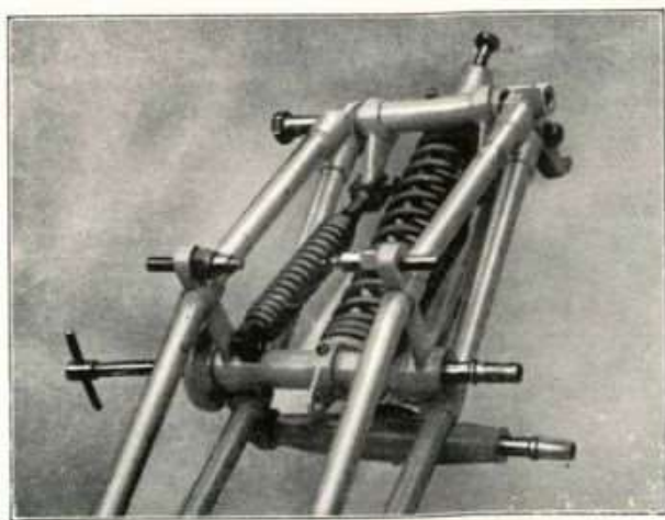
Fig. 34 - Come si levano i perni inferiori.
