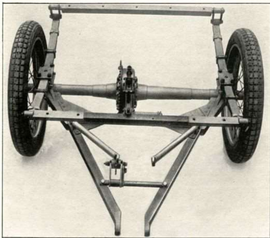
Fig. 98 - Telaio porta-cassone completo.
