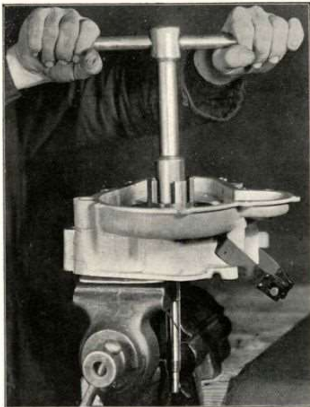
Fig. 50 - Come si prende in morsa l'albero primario del cambio e si smontano il controdado e dado di bloccaggio del corpo frizione fisso (griffa).
