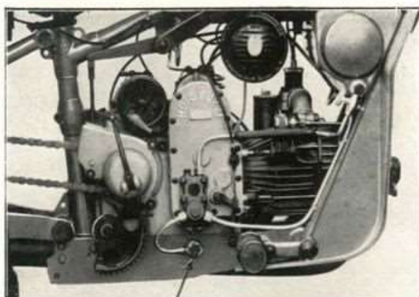
Fig. 97 - È visibile il diverso piazzamento del tubo ricupero, olio (confrontare fig. 15).
