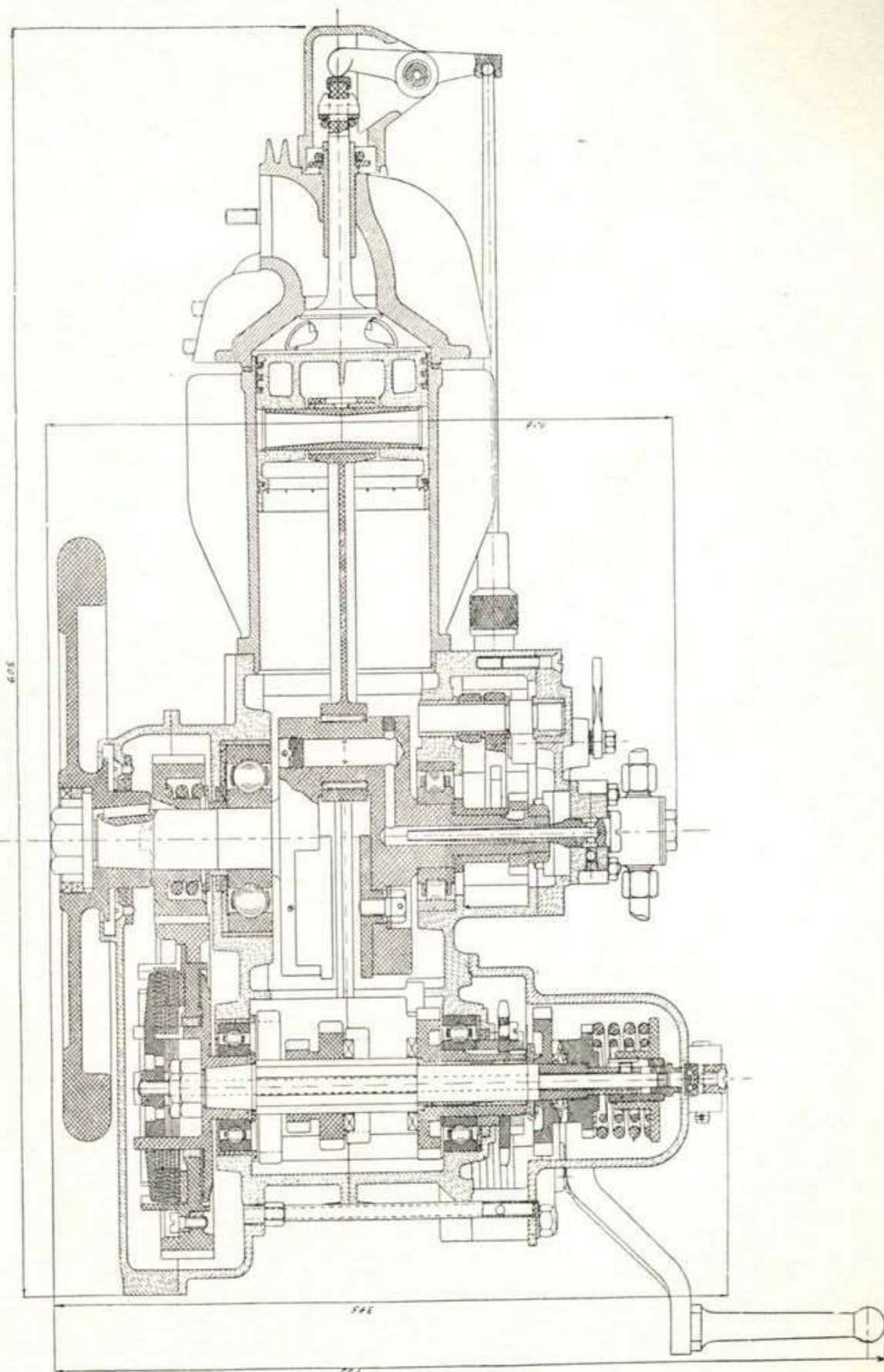
Sezione longitudinale orizzontale del motore.
