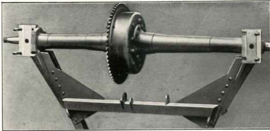
Fig. 99 - Gruppo differenziale visto dall'alto. Si notino i 4 bulloni esterni di fissaggio delle balestre.
