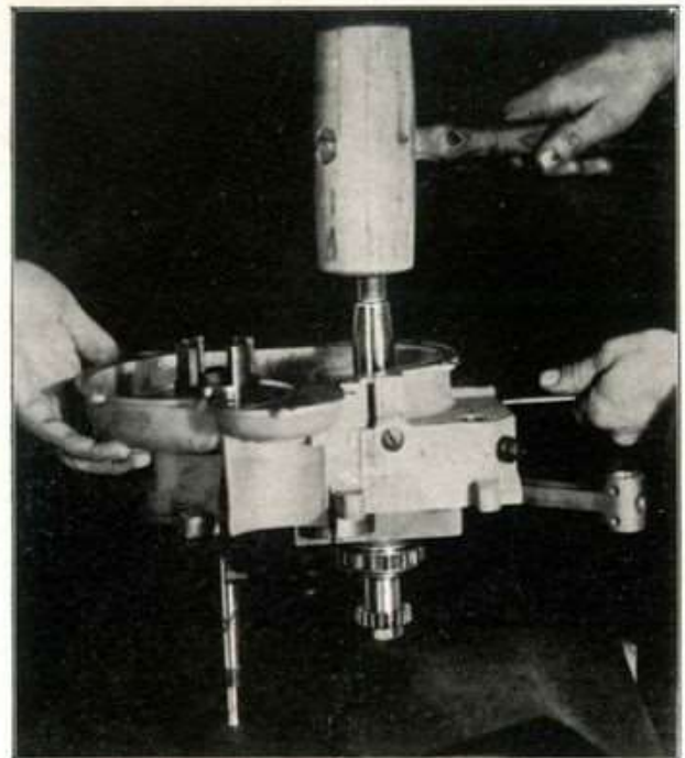
Fig. 48 - Come si leva il gruppo albero a gomito biella. Tenendo sospeso il mezzo carter e battendo dall'esterno verso l'interno.
