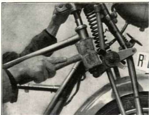
Fig. 29 - Come si sfila il canotto di guida dalla testa di sterzo.
