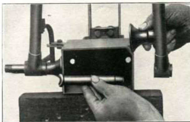
Fig. 32 - Come si levano i due mezzi perni e i rocchetti spessore.
