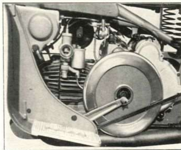
Fig. 4 - Motore montato sul telaio, lato volante.
