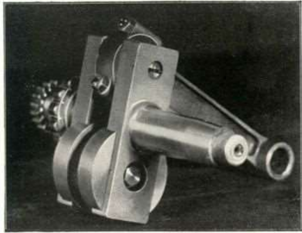
Fig. 57 - Albero a gomito biella visto dal lato volano. Si noti il tappo di ispezione per canale interno dell'olio.
