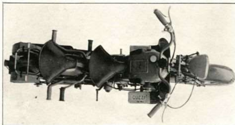
Fig. 6 - Si noti la disposizione dei comandi.
