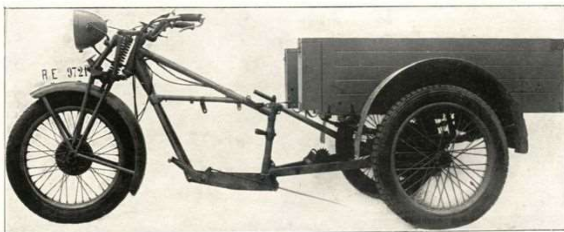
Fig. 95 - Moto telaio 32, vista senza motore.
