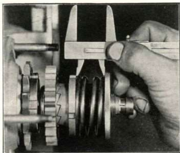
Fig. 62 - Come si regola la tensione delle molle della frizione. La misura normale, come indicato in figura, è mm. 28.
