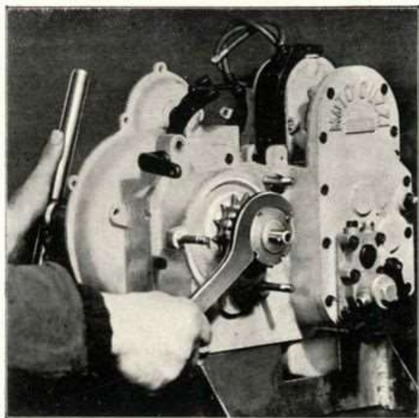
Fig. 43 - Come si smonta il manicotto dentato per la messa in moto.
