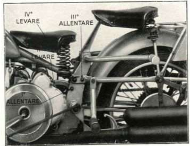
Fig. 17 - Le ultime operazioni da eseguirsi per aprire il telaio e togliere il motore.
