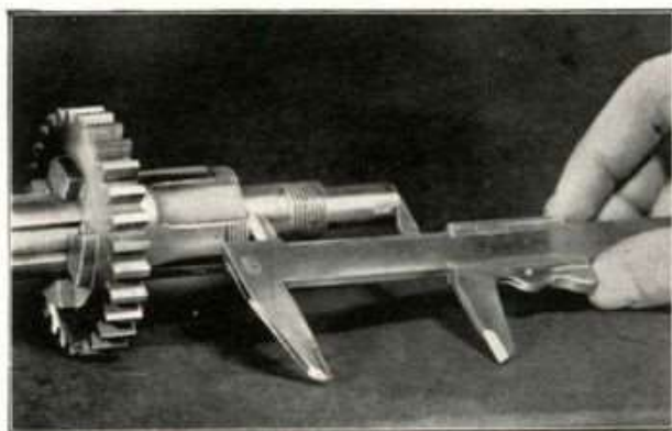
Fig. 63 - Come si misura la distanza fra l'estremità destra dell'albero primario e l'estremità destra dell'ingranaggio presa diretta.
