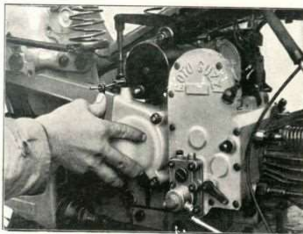
Fig. 14 - Come si smonta il comando della frizione.
