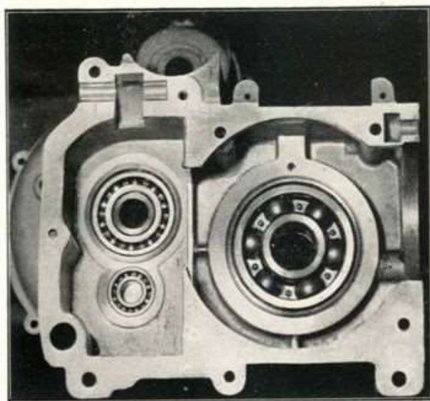
Fig. 49 - Vista interna del mezzo carter sinistro (lato volano). Si notino il cuscinetto a sfere (grande) per albero motore, il cuscinetto piccolo per albero secondario cambio e il cuscinetto per albero primario. Si noti che in quest'ultimo è ancora montato il corpo frizione fisso (anello interno) che si estrae battendo dall'interno verso l'esterno sull'albero cavo (conico).
