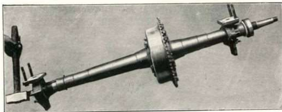
Fig. 103 - Battendo sul semiasse sinistro si è ottenuto il distacco dell'anello interno del cuscinetto sinistro. Si noti la fuori uscita del cuscinetto destro.
