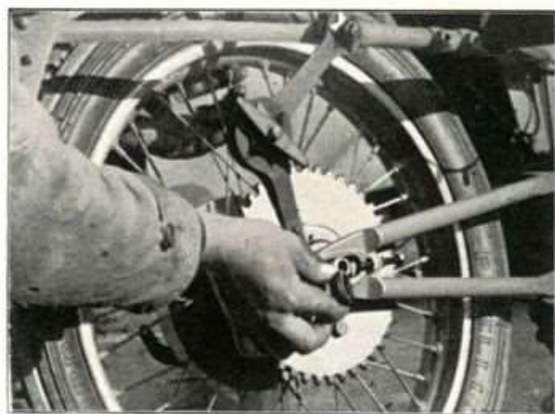
Fig. 20 - Come si leva la ruota posteriore - Il perno è già stato sfilato - Si vede nella mano il dado per perno forato.
