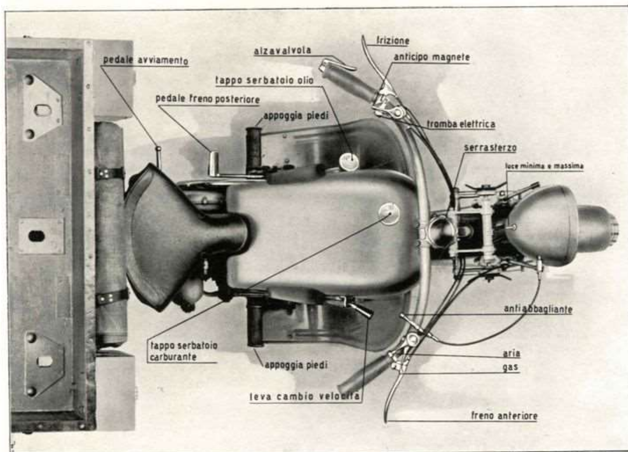
Fig. 93 - Mototriciclo 32, comandi.
