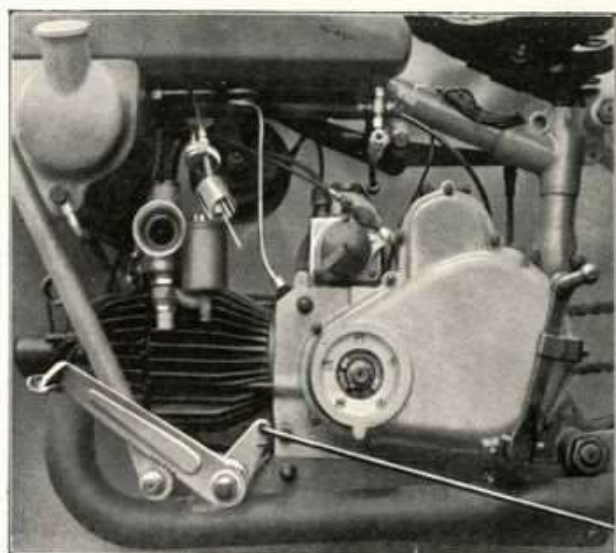
Fig. 96 - Si notino: le valvole di regolazione gas e aria estratte dal carburatore; la posizione del pedale del freno. Il tubo sfiatatoio dell'olio e i due bulloni che uniscono telaio porta motore e telaio porta cassone.
