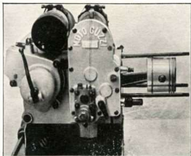
Fig. 38 - Motore senza cilindro e testa.
