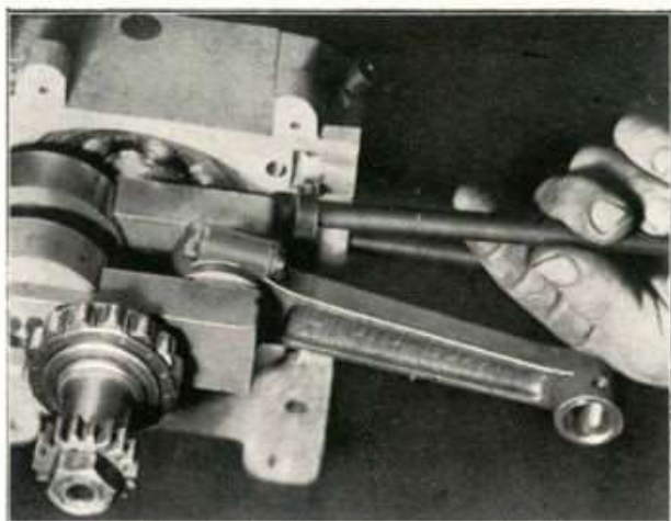
Fig. 75 - Prima di chiudere i due mezzi carter ricordare di piazzare il tirante per fissaggio testa e cilindro.
