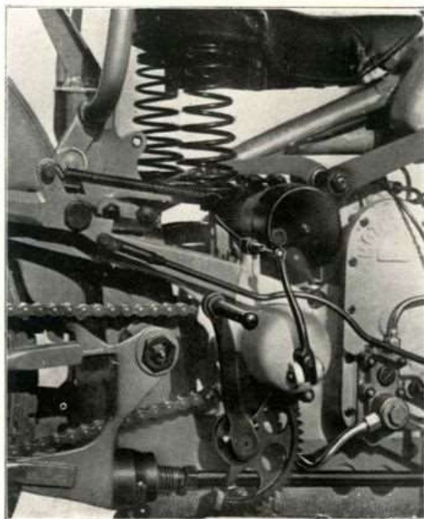
Fig. 10 - Moto biposto - Gruppo frizione - Avviamento Pompa olio. Sono visibili in basso i tiranti del forcellone oscillante.
