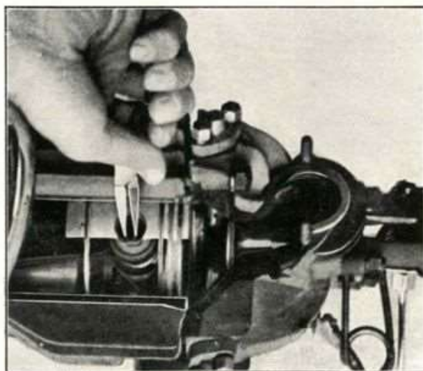
Fig. 39 - Come si leva la molletta (sinistra) che fissa lo spinotto. (Il motore è sezionato).
