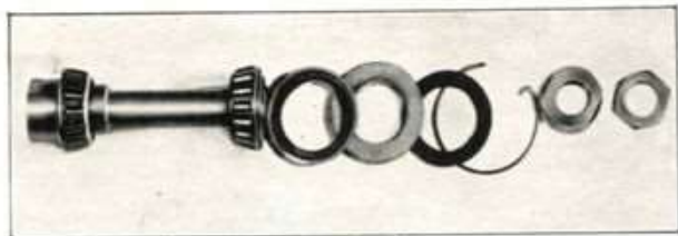
Fig. 87 - Mozzo anteriore. Ordine di montaggio dei vari pezzi.
