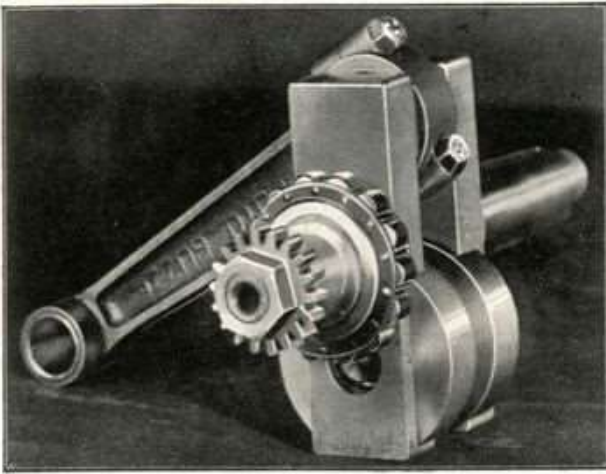
Fig. 56 - Gruppo albero a gomito biella visto dal lato distribuzione. Si notino il dado smussato all'esterno e la bulinatura di sicurezza.
