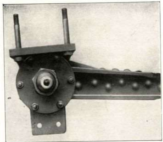
Fig. 101 - Supporto per molle a balestra destra. Si notino i 6 bulloni di chiusura del coperchio, il dado manicotto di serraggio del cuscinetto e i 2 bulloni esterni di fissaggio della balestra.
