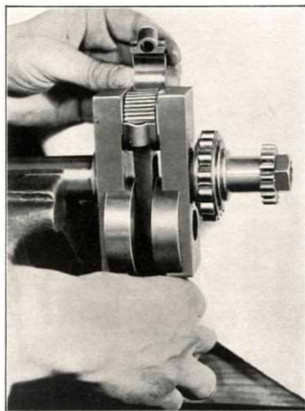
Fig. 59 - Come si montano i rullini della biella.
