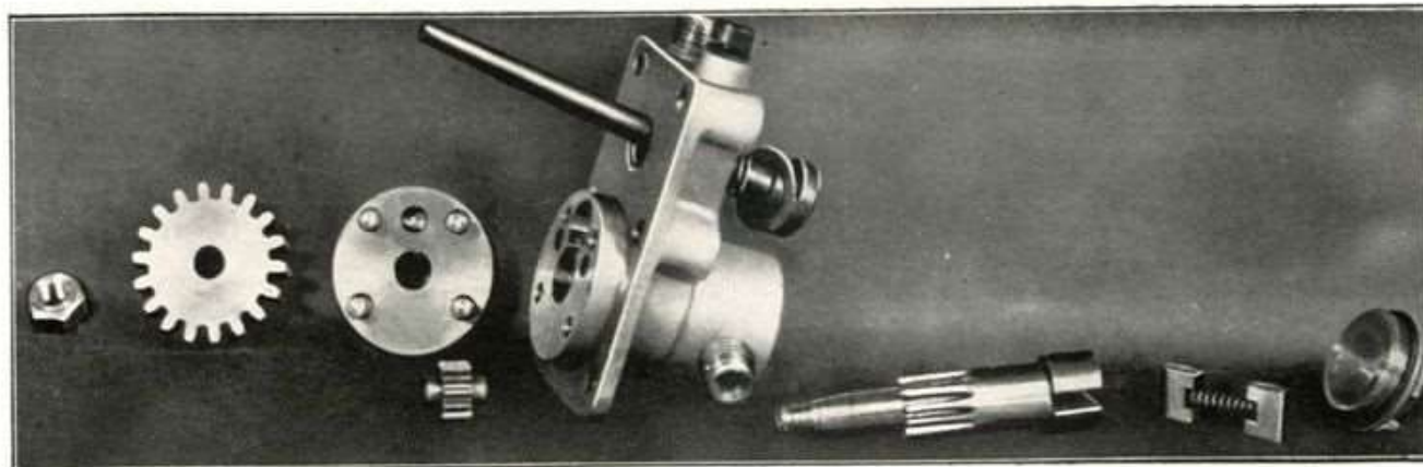
Fig. 70 - La pompa dell'olio smontata. Ordine di montaggio dei singoli pezzi.
