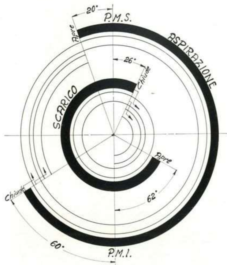
Diagramma angolare di distribuzione riferito all'asse motore
