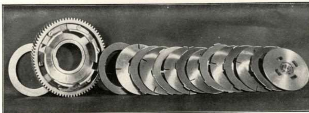
Fig. 61 - (da sinistra a destra - dall'interno all'esterno). Ordine di montaggio dei vari pezzi costituenti la frizione.
