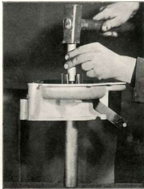
Fig. 51 - Dopo avere infilato sull'albero primario un tubo di ferro, ecco come si sfila l'albero medesimo.
