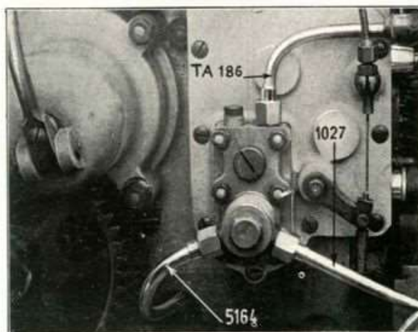
Fig. 15 - Vista della pompa olio e dei tre raccordi: Superiore - Anteriore - Posteriore.
