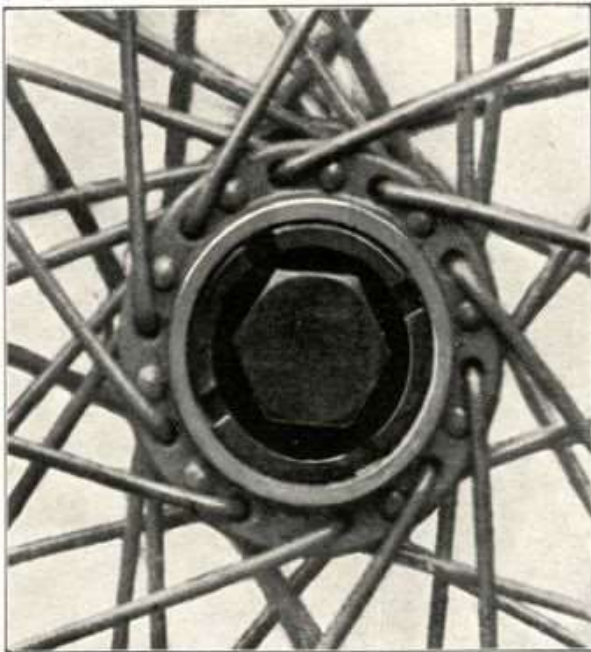
Fig. 100 - Particolare ruota posteriore del mototriciclo. Si noti l'anello controdato (filetto sinistrorso) e il dado interno (filetto normale destro).
