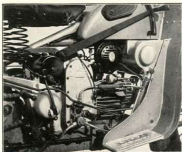
Fig. 3 - Motore montato sul telaio, lato distribuzione.
