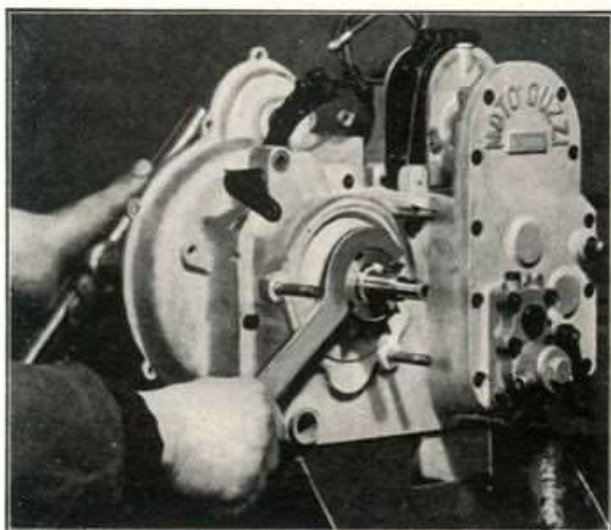
Fig. 44 - Come si smonta la ghiera di serraggio del pignone del cambio.
