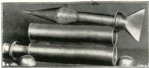
Fig. 68 - Come è formato il silenziatore nelle moto mono e biposto.
