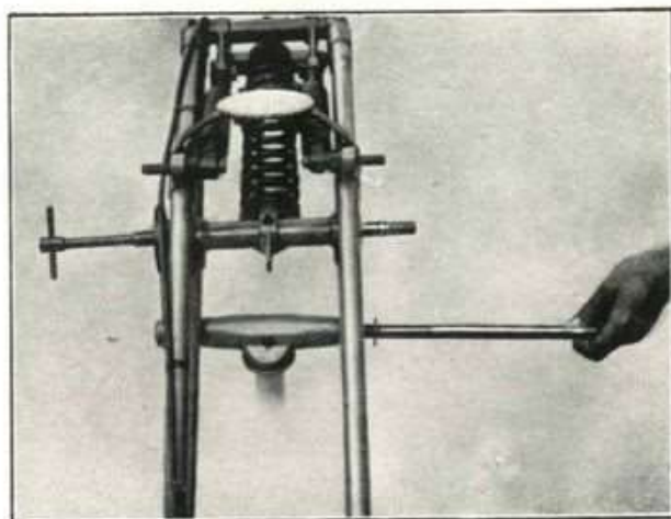
Fig. 35 - Come si levano i perni inferiori. Avvitare completamente e sfilare a sinistra.
