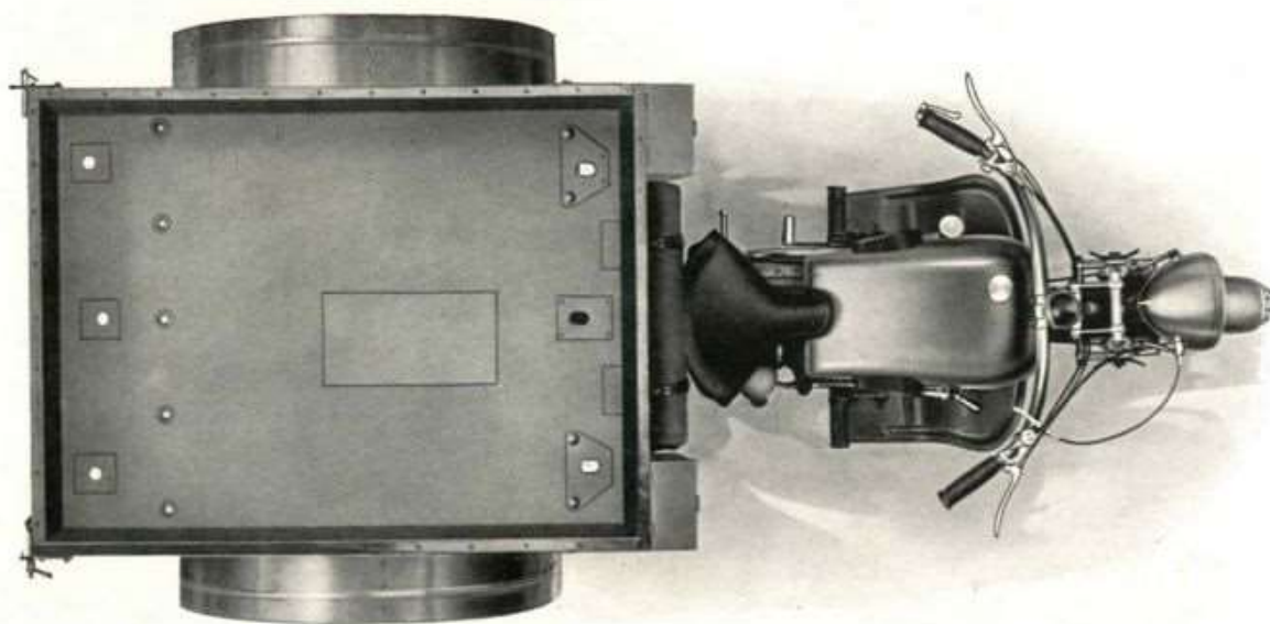
Fig. 92 - Mototriciclo 32, vista in pianta.
