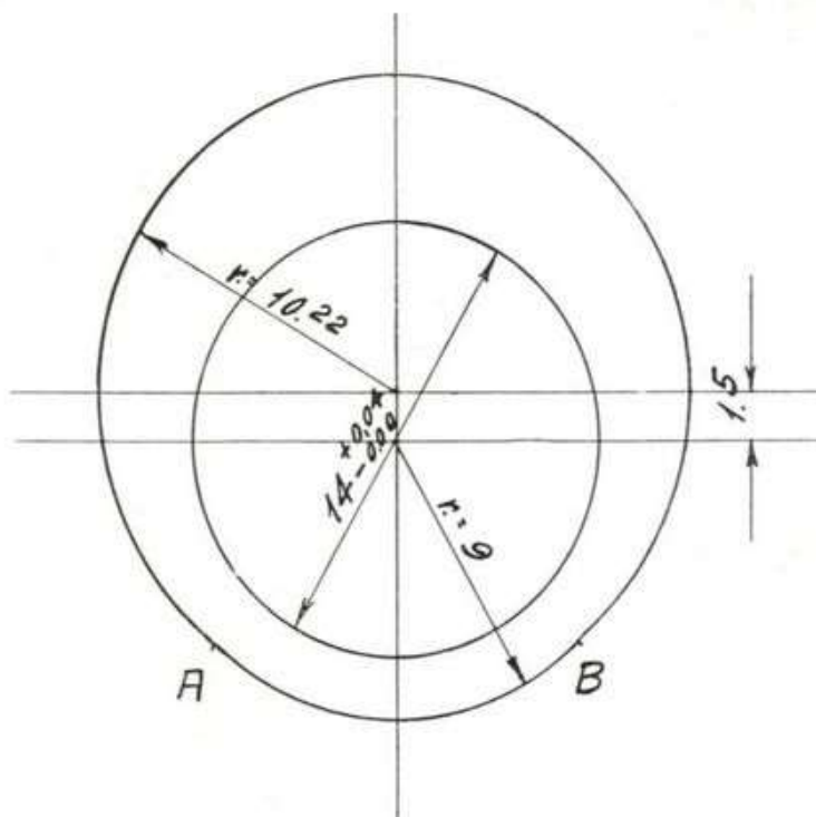
Fig. 73 - Schema sede delle palette.
