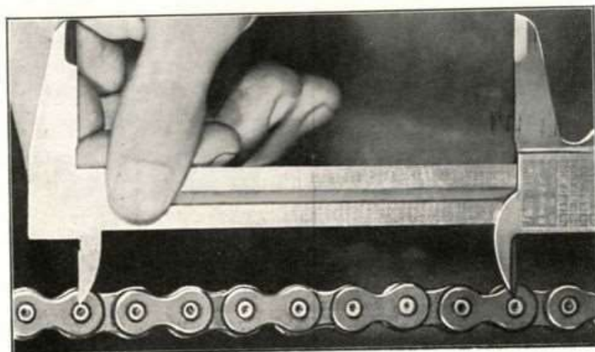
Fig. 66 - Come si controlla l'allungamento della catena di trasmissione.
