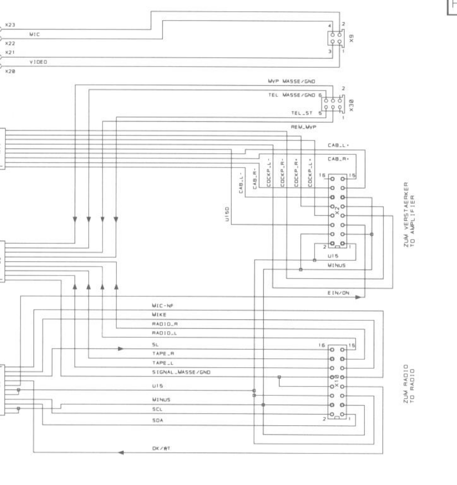
ANSCHLUSSPLATTE CONNECTOR-PCB
