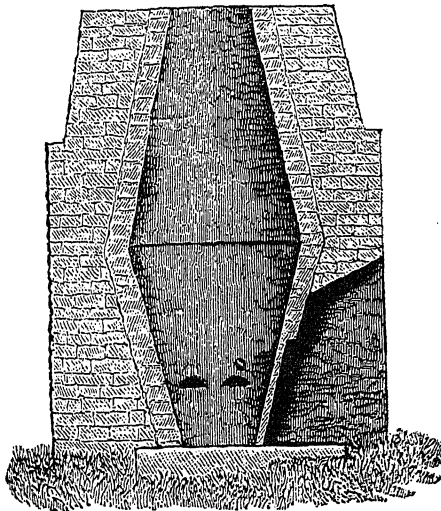
Fig. 1.—German Stückofen.
