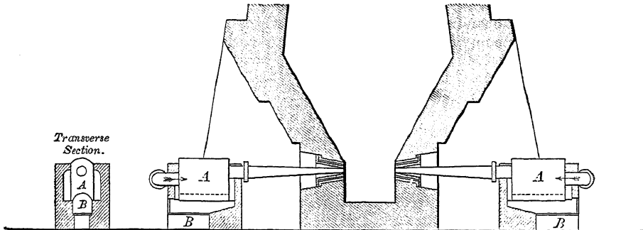
Fig. 5.—Neilson's original hot blast apparatus, 1829.
