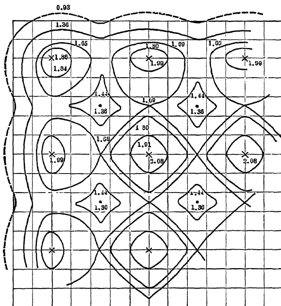
FIG. 76.—Illumination contours.
