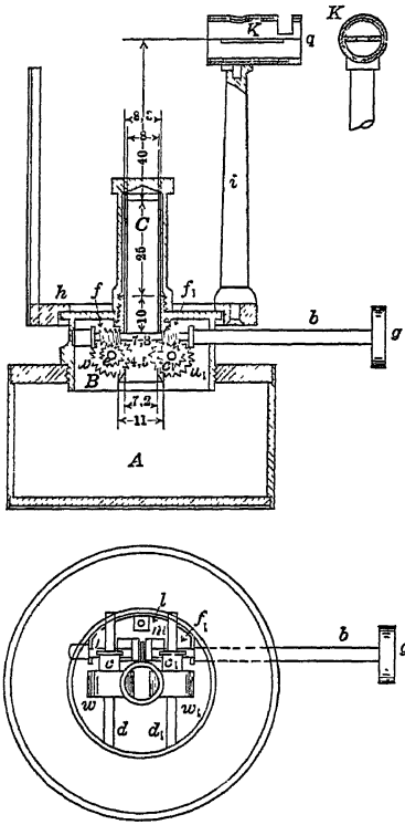
FIG. 42.—Hefner lamp.
