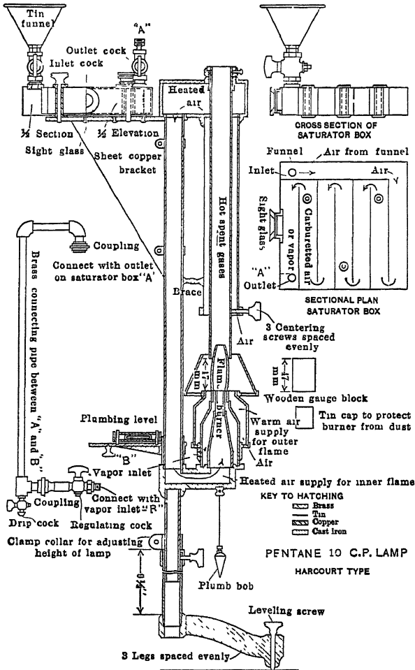
FIG. 41.—Harcourt pentane lamp.
